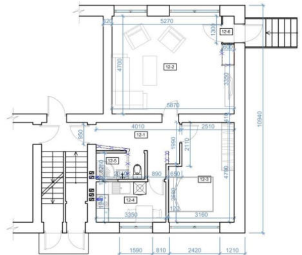
PATALPOS PATALPŲ PLANAS PO REMONTOS IR PASKIRTIE KEITIMO PAKEITIMO M1:100
