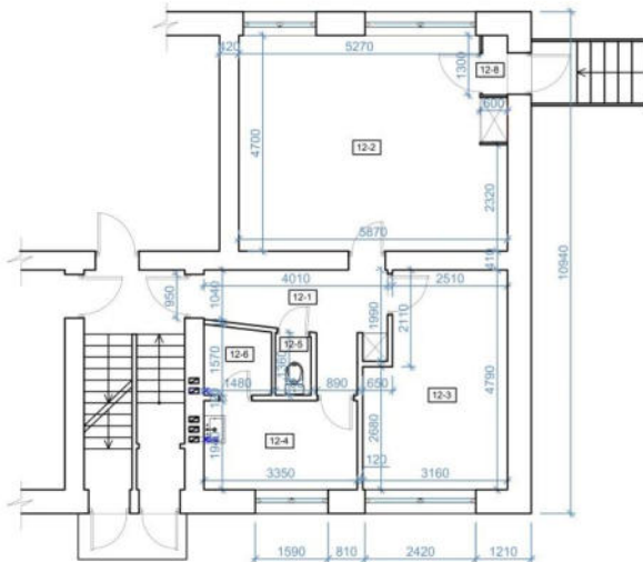
PATALPOS PATALPŲ PLANAS IKI REMONTOS IR PASKIRTIE KEITIMO PAKEITIMO M1:100
