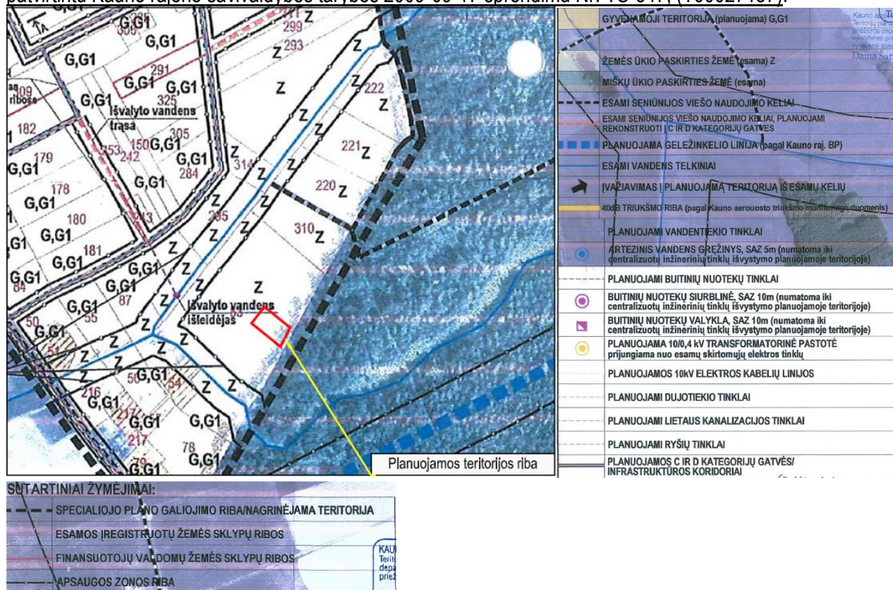
5 pav. Ištrauka iš Gyvenamųjų namų ar kitos paskirties pastatų ir statinių teritorijų išdėstymo Kauno r. sav., Karmėlavos sen., Sergeičikų I kaimo dalies teritorijos, apimančios Karmėlavos kadastrinės vietovės 13 bloko dalį, specialiojo plano.
